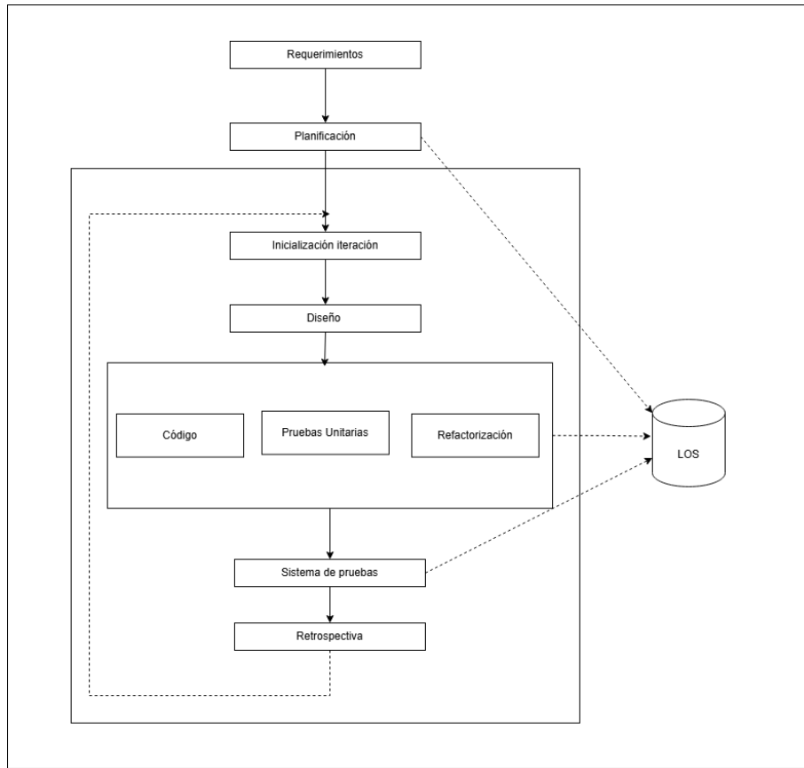
Figura 2.1: Fases de metodología Personal Extreme Programming (PXP).
