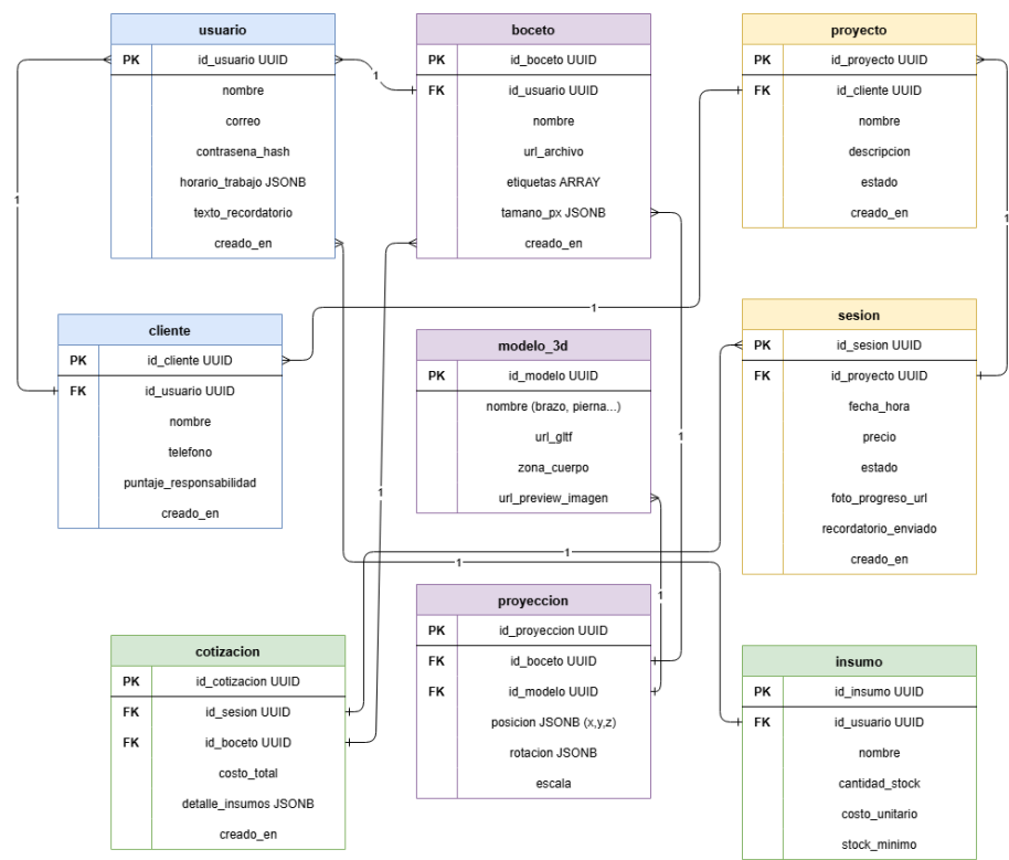
Figura 4.3: Diagrama Entidad-Relación del modelo de datos del sistema.
