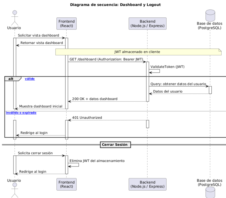
Figura 4.13: Diagrama de secuencia HU02: Dashboard.
