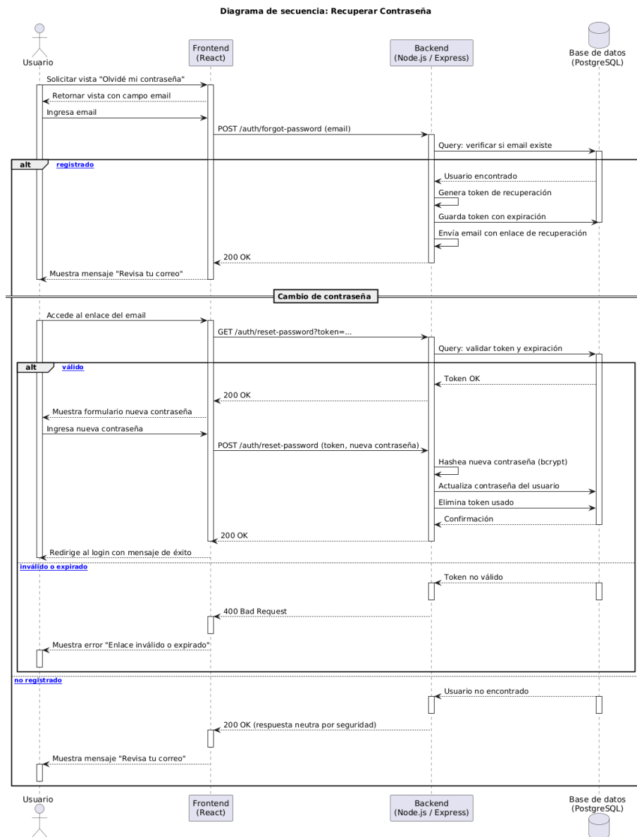
Figura 4.14: Diagrama de secuencia HU03: Olvidar Contraseña.
