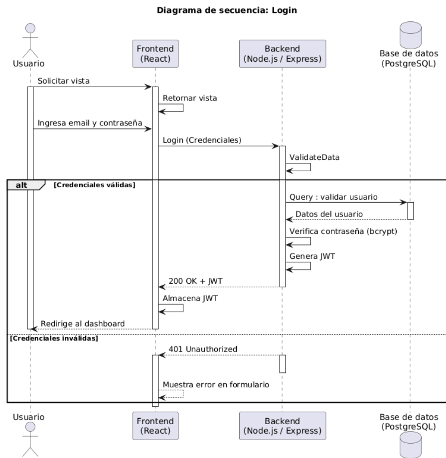
Figura 4.12: Diagrama de secuencia HU01: Login.
