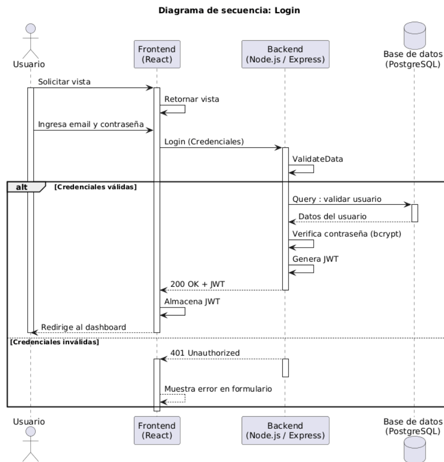
Figura 3.2: Ejemplo de diagrama de secuencia para el inicio de sesión.
