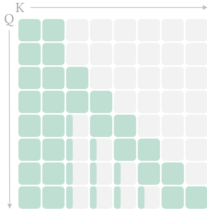
Geometric Context Attention (d)
