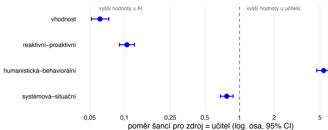
Obrázek 4: Obrázek 7.4. Citlivostní CLMM: poměry šancí pro zdroj = učitel na logaritmické ose (95% Waldovy intervaly spolehlivosti; svislice OR = 1 značí žádný rozdíl mezi zdroji; hodnoty viz Tabulka 7.2). Zdroj: manifest kap7_k2_shoda_cisla.csv (skript fig_07_hloubka.R ).
