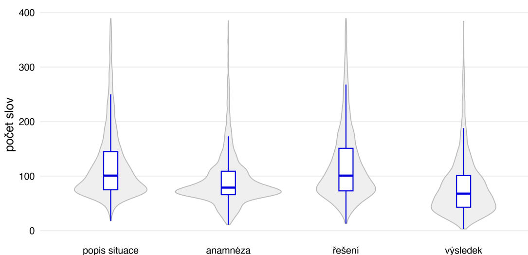
Obrázek 2: Obrázek 5.2. Rozdělení délek čtyř částí kazuistiky (počet slov; houslový graf s vytyčeným mezikvartilovým rozpětím a mediánem; pro čitelnost oříznuto na 99. percentil). Zdroj: kap5_delky_rozdeleni.csv (notebook 10_korpus.qmd , skript fig_05_hloubka.R ).
