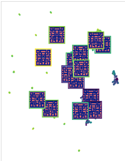
CLIP
