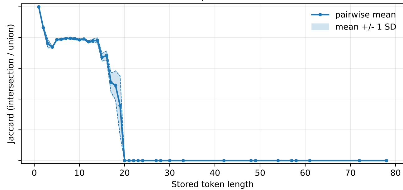
bpe
