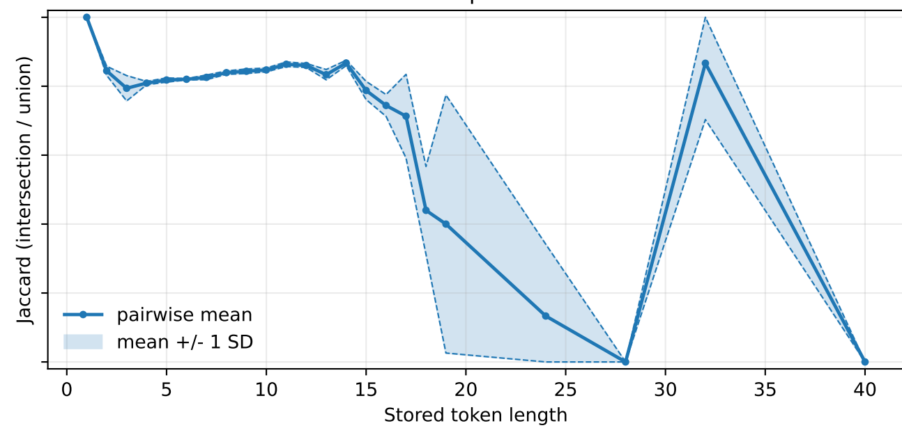
bpe
