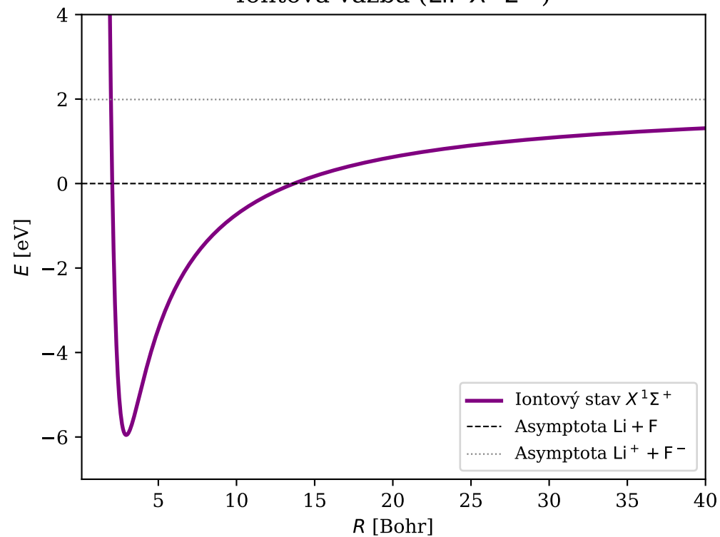
Iontová vazba ( \text{LiF} \ X^1\Sigma^+ )
