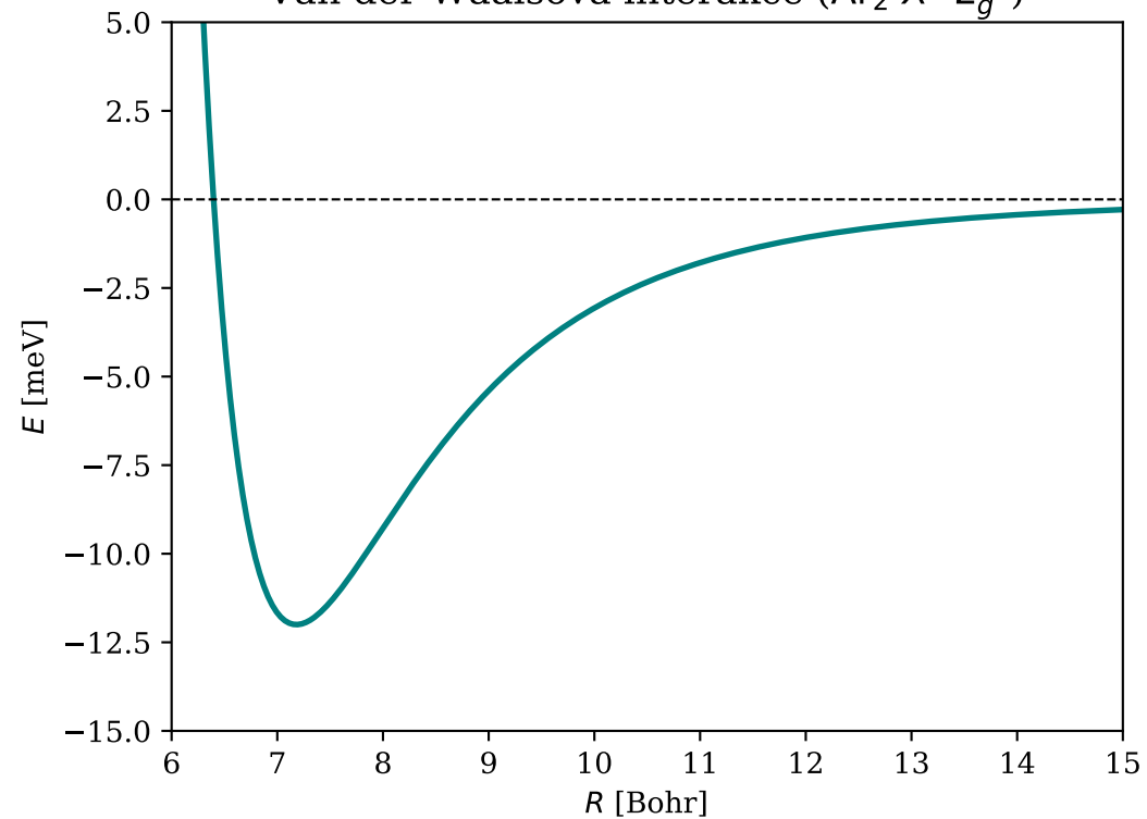
Van der Waalsova interakce ( \text{Ar}_2 \ X^1\Sigma_g^+ )
