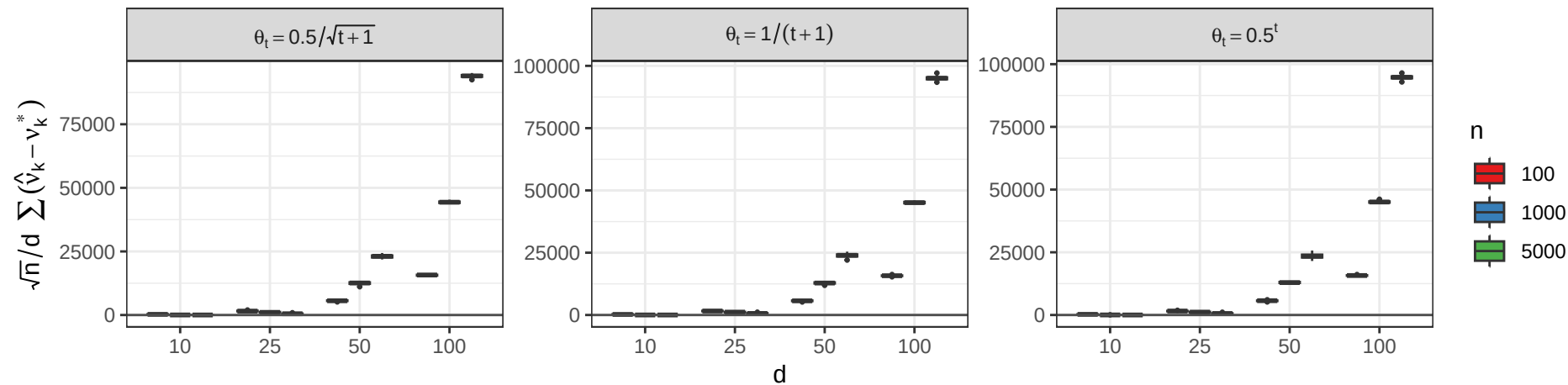
C-Vine
