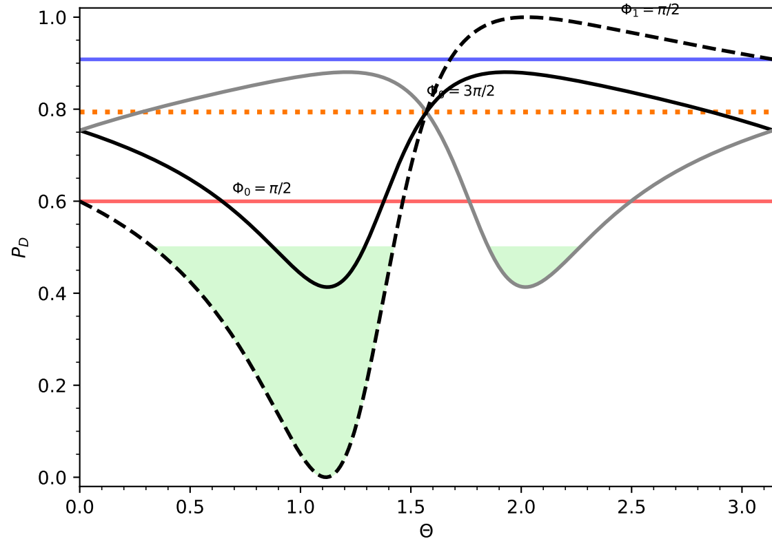
dCNOT (++)
