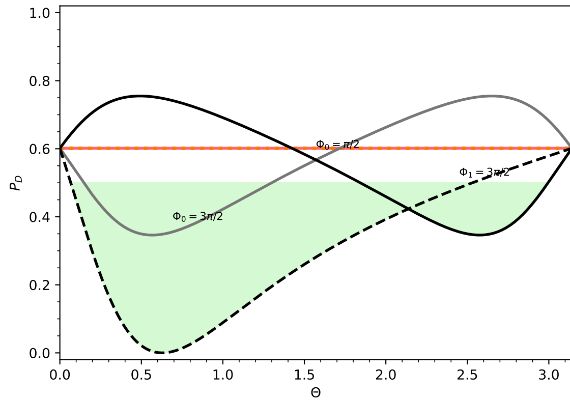
CNOT (++)
