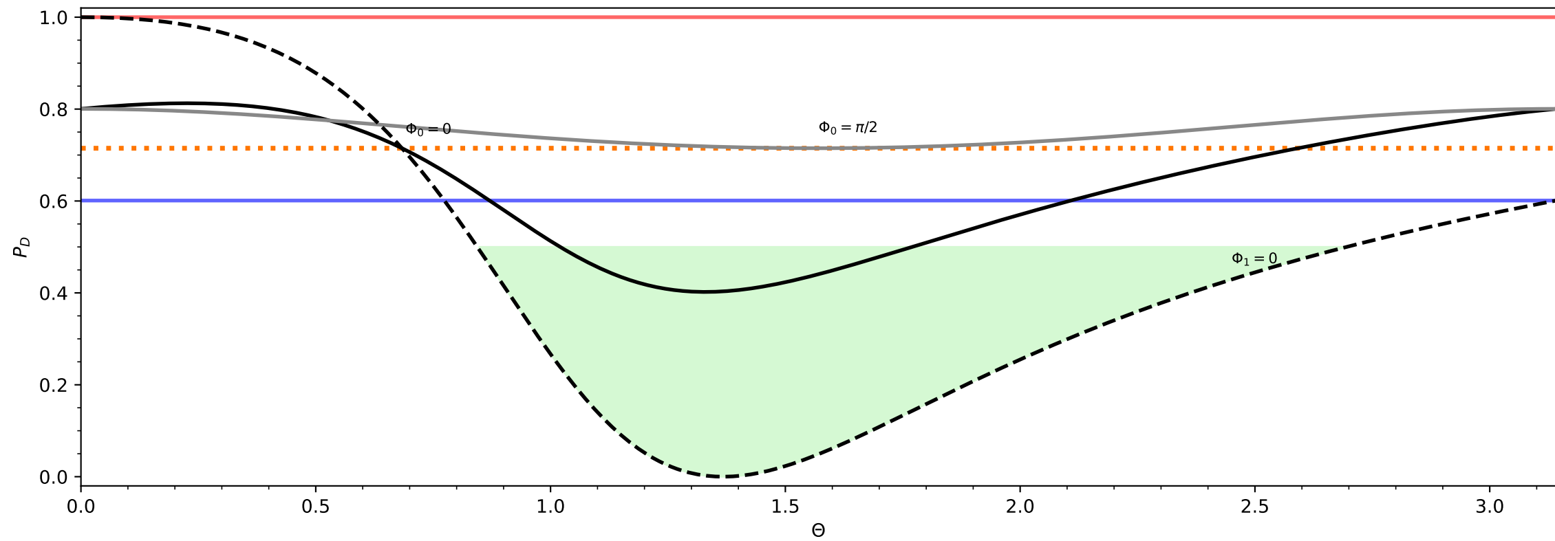
dCNOT (++)
