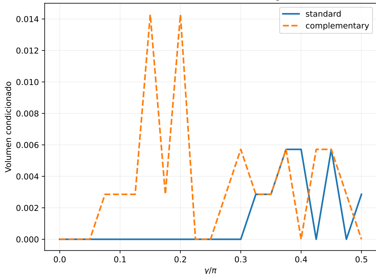
Entrelazamiento crítico (EWL original)
