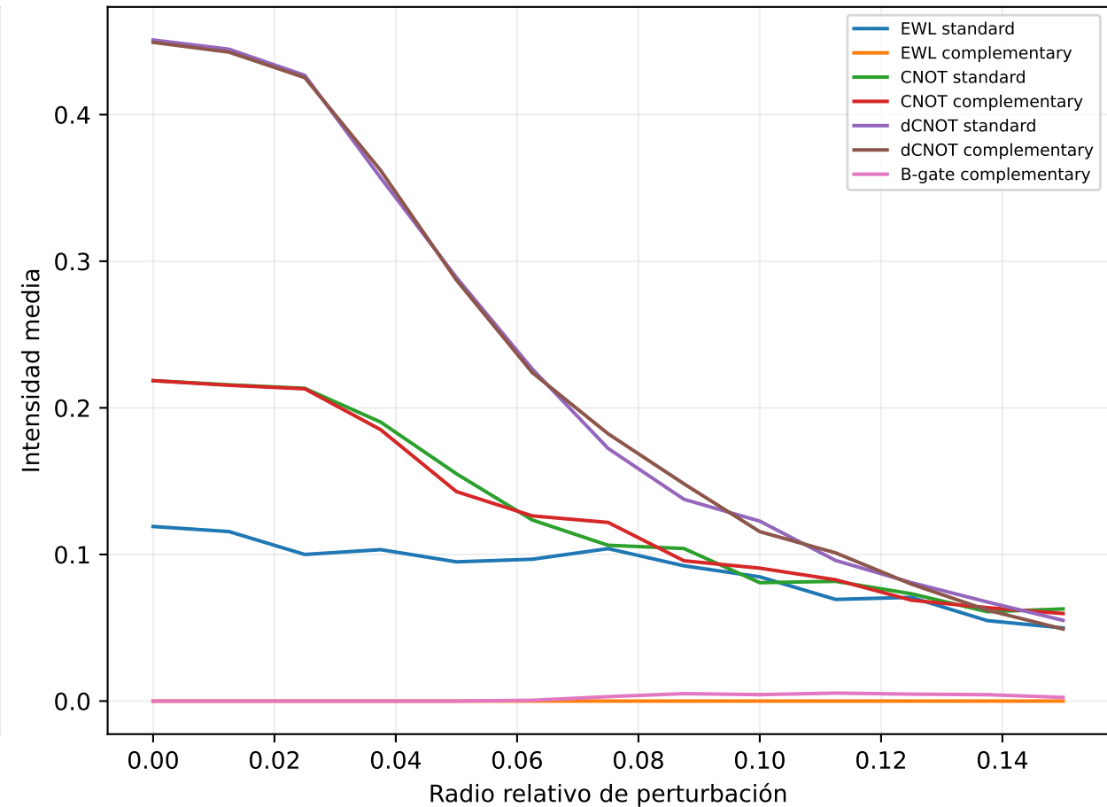
Degradación de la intensidad
