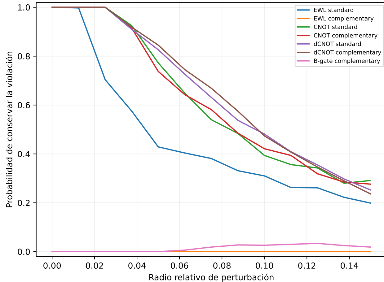
Robustez de la región violatoria
