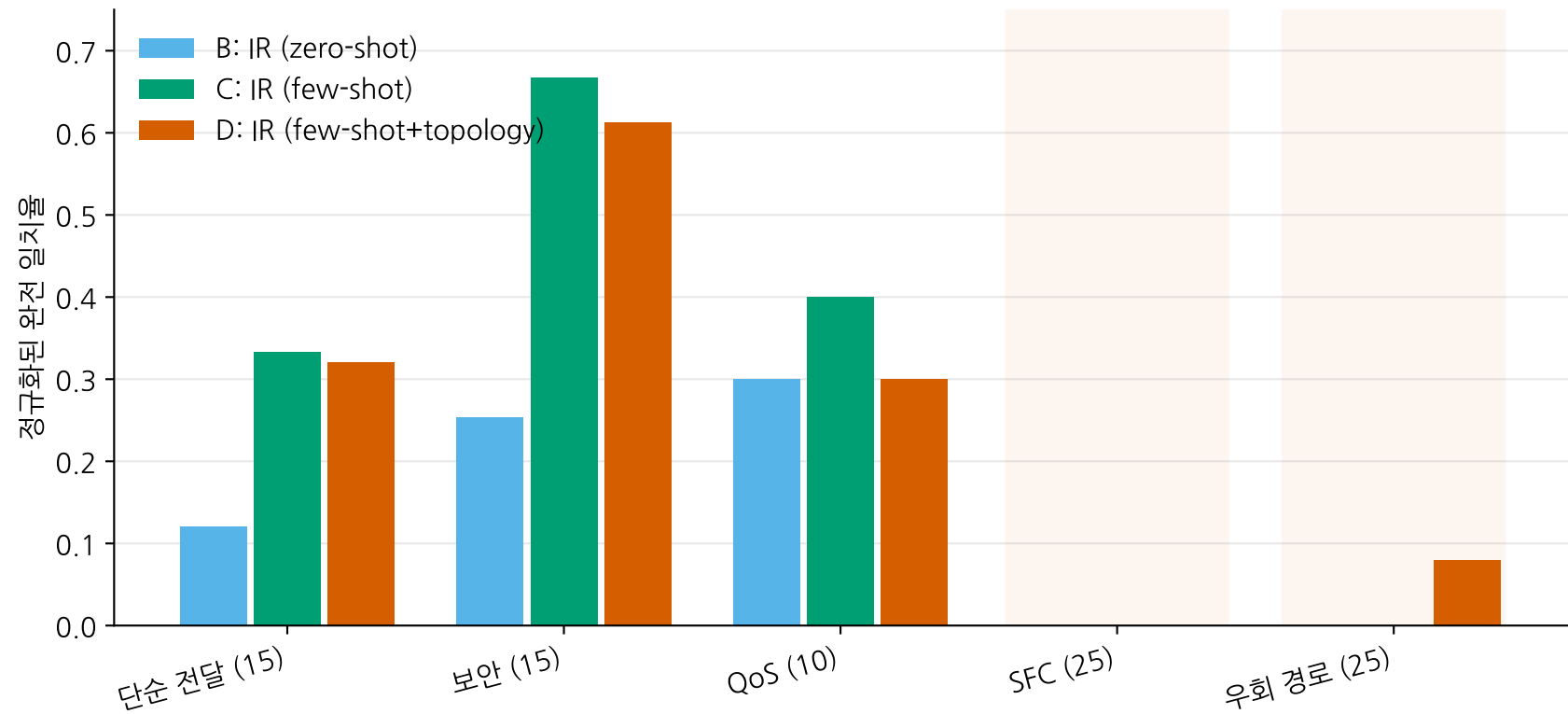
SFC/우회 확장: 기존 카테고리는 개선되지만 SFC는 0%로 붕괴
