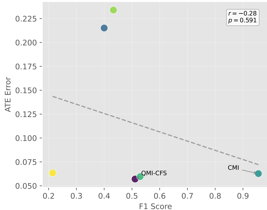
IHDP: F1 vs. ATE Error
