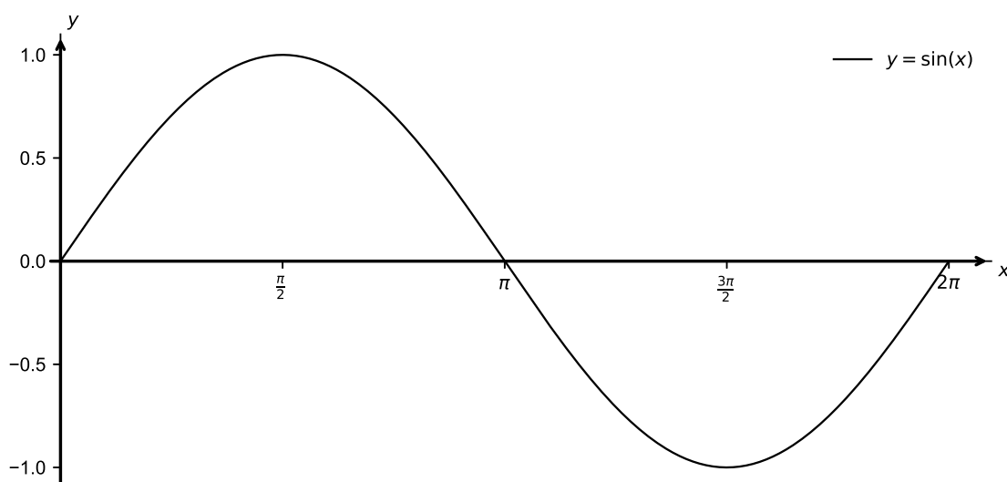
Rys. 3.1. Wykres funkcji sinus. Kod programu w Pythonie wykres znajduje się w Dodatku A.
