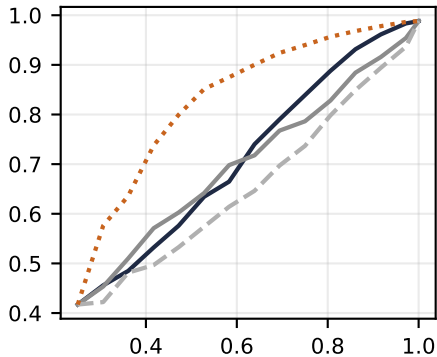
Cu
