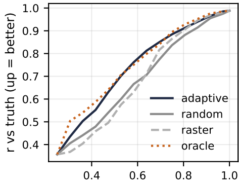
Ca
