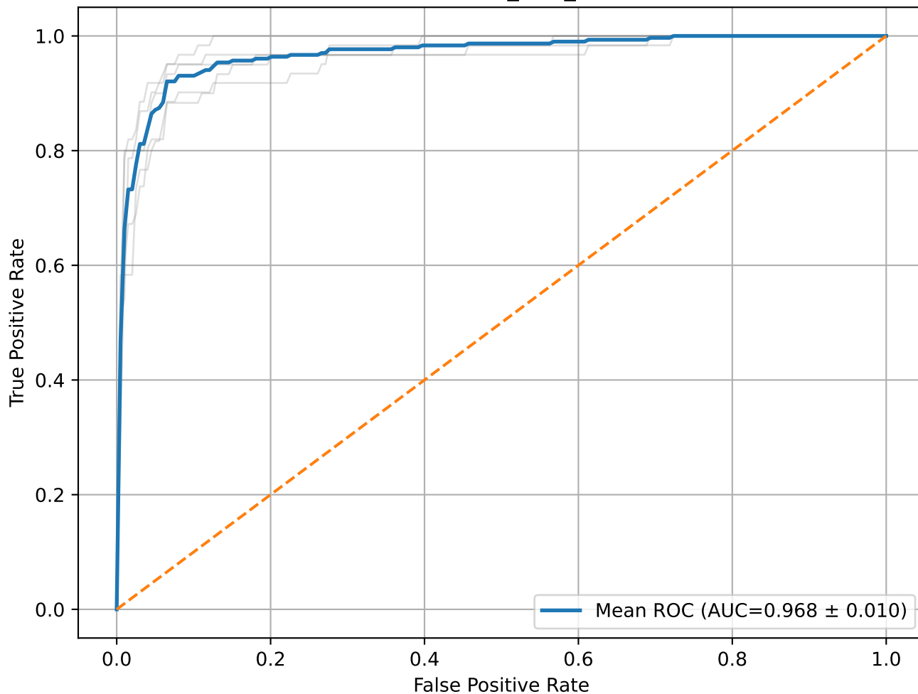
ROC - BAYES_OPT_SVMS
