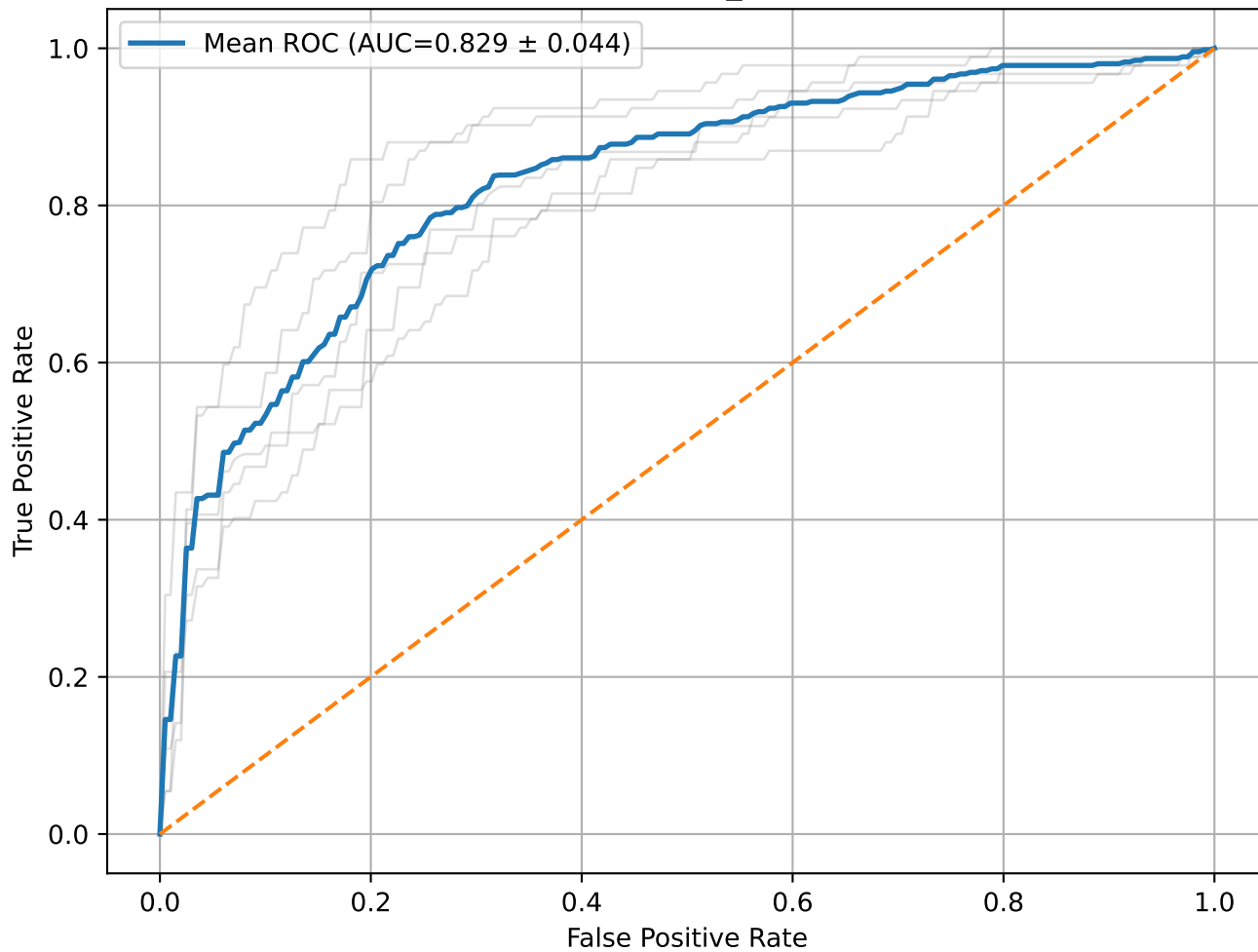
ROC - PSO_SVM
