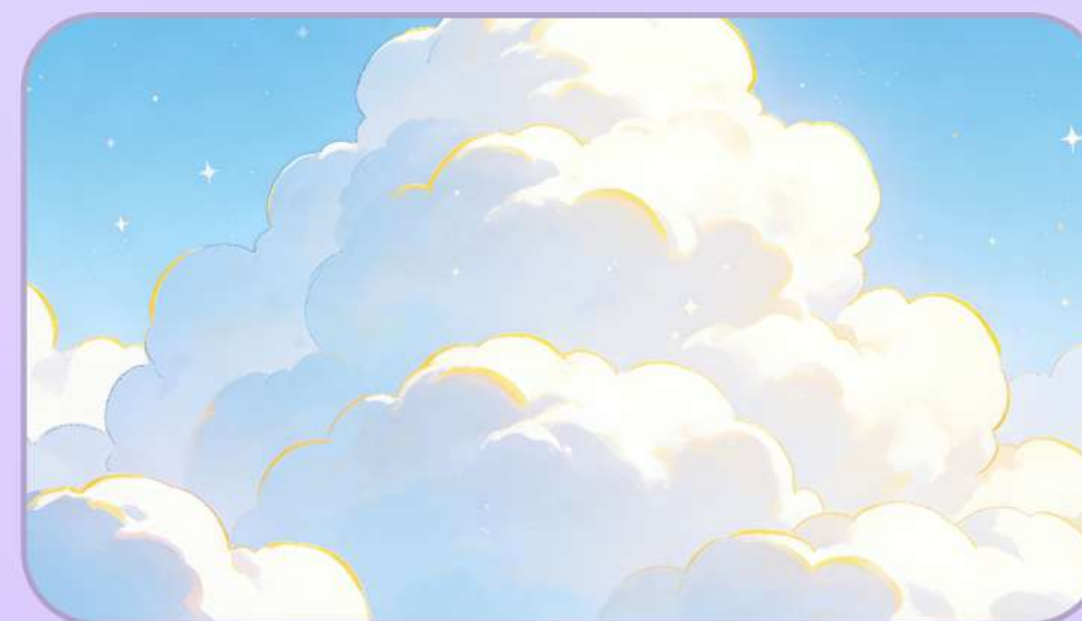
云层
