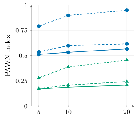
(d) p_0 = 10\%
