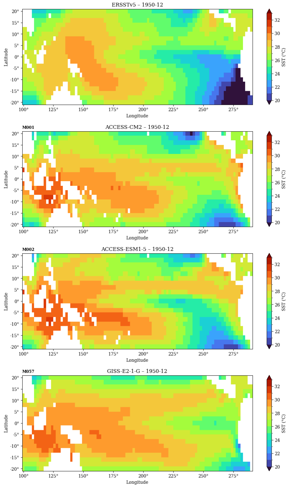
Figura 5: Comparación espacial de la temperatura superficial del mar media del periodo histórico común (mes de muestra 1950-12), ya en la grilla, calendario, unidades y máscara océano-tierra homogeneizados por el pipeline (Pasos 04–05). De arriba hacia abajo: observado (ERSSTv5) y los tres modelos de grilla nativa más gruesa entre los seleccionados – cada panel indica su propia fuente/identificador M001–M102 (Cuadro 3) directamente en el título del gráfico; esta figura es una verificación visual de que dicha condición se cumple incluso en el caso más exigente (grilla nativa más gruesa), no un resultado de desempeño.
