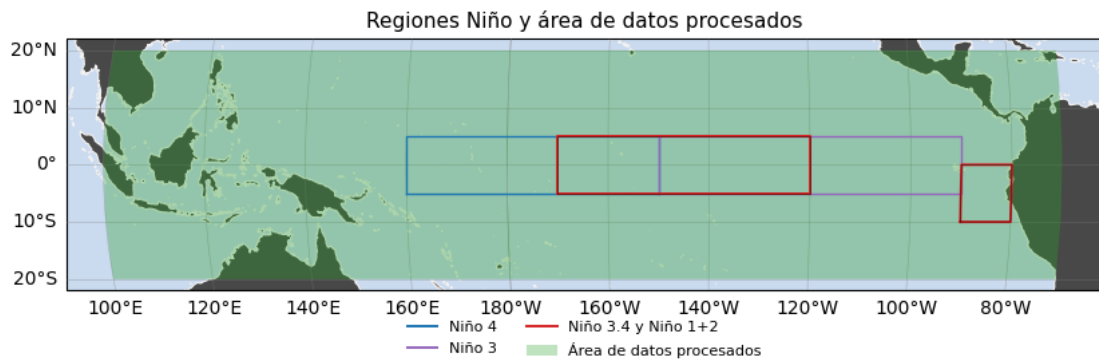
Figura 2: Regiones oceanográficas Niño 3.4 ( 170^\circ\text{O} – 120^\circ\text{O} , 5^\circ\text{S} – 5^\circ\text{N} ) y Niño 1+2 ( 90^\circ\text{O} – 80^\circ\text{O} , 10^\circ\text{S} – 0^\circ , ambas con doble borde en la figura) sobre el Pacífico tropical oriental, en proyección Robinson centrada dinámicamente en el punto medio de Niño 3.4 ( config/domains.yaml ). El área verde es la ventana de descarga real ( 100^\circ\text{E} – 70^\circ\text{O} , 20^\circ\text{S} – 20^\circ\text{N} , Sección 4.3): todo el dominio efectivamente descargado, regrillado y enmascarado por el pipeline . Niño 1+2, adyacente a la costa peruana y a la zona de surgencia de la Corriente de Humboldt, es la caja de mayor relevancia directa para el monitoreo del Niño costero en Perú (Takahashi and Martínez, 2019), mientras que Niño 3.4 es la caja estándar internacional del Índice Oceánico de El Niño (ONI).
