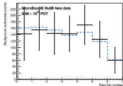
p_\mu
