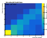
p_n
