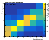
W_{had}
