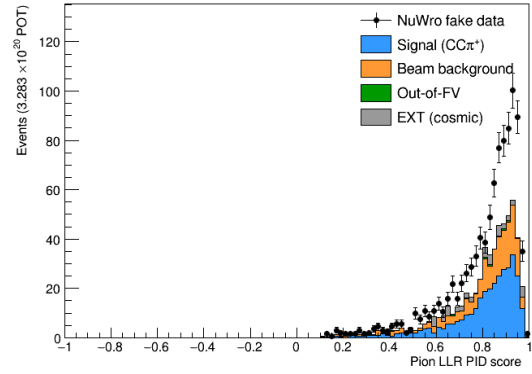
(d) Pion LLR PID.
