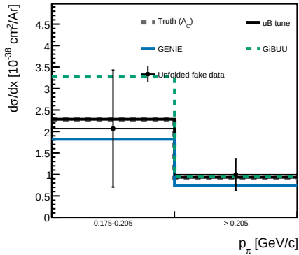
ppi
