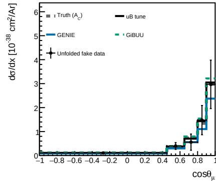
costhmu
