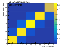
\theta_{\mu\pi}
