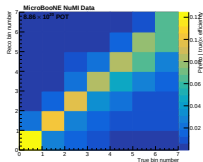
p_\mu
