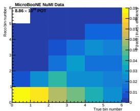
W_{\pi p}
