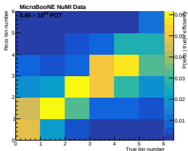
W_{had}
