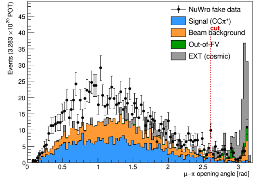
(d) \mu - \pi opening angle (Cut 9).
