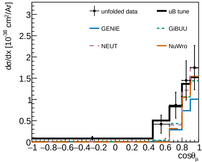
costhmu ( A_C -smeared)
