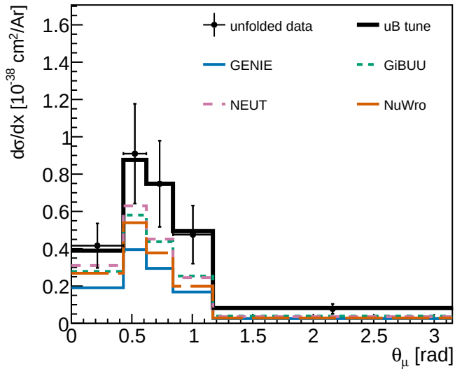
thetamu ( A_C -smeared)
