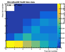
W_{\pi\rho}
