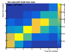
W_{had}
