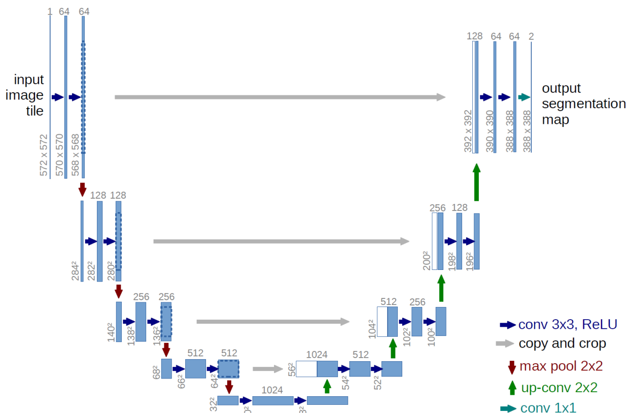
Obrázek 4.1.: Architektura U-Net sítě dle Ronneberger et al. [21]
