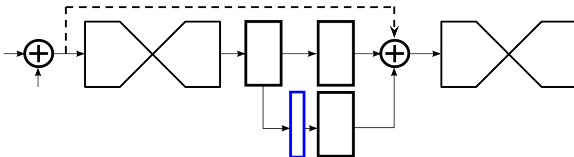
Obrázek 4.2.: Schématické znázornění architektury stacked hourglass network dle Newell et al. [28]
