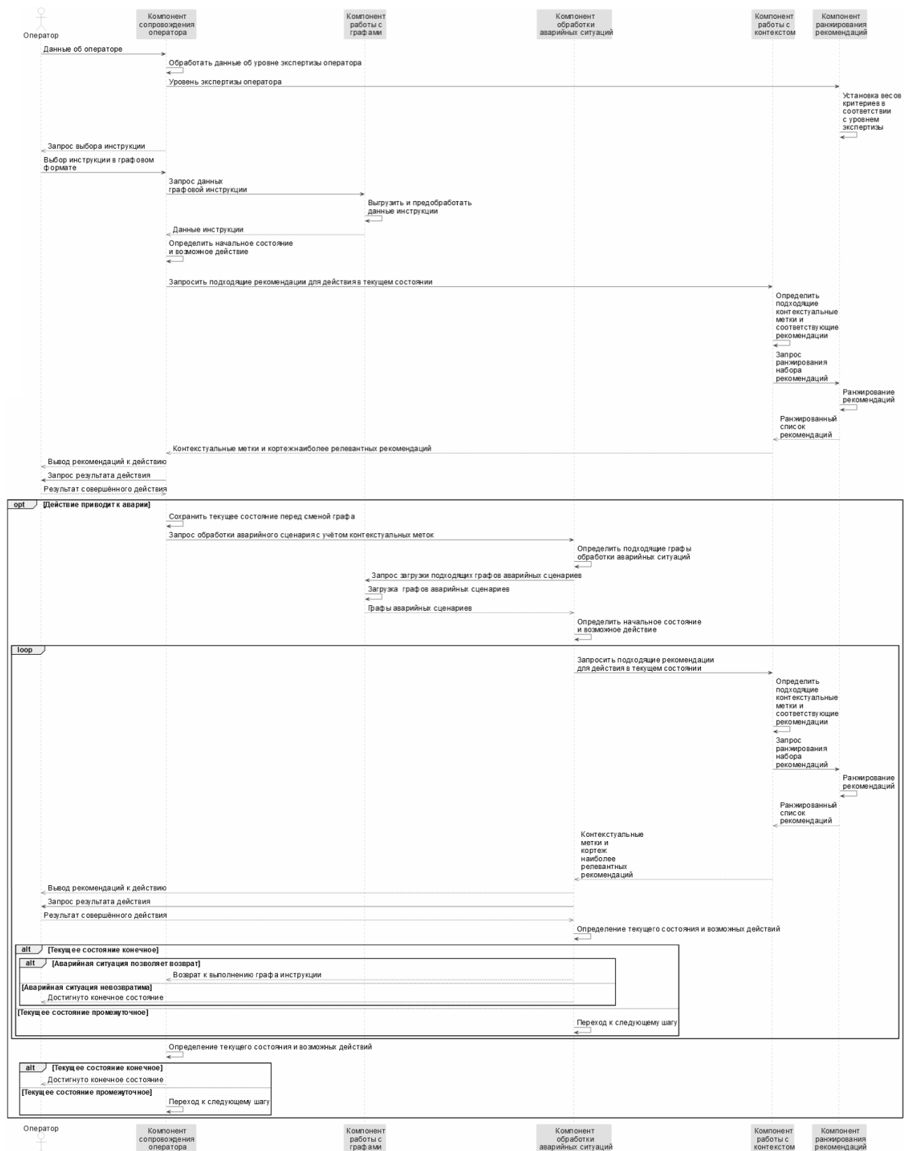
Рисунок 2.8 – Диаграмма последовательности
