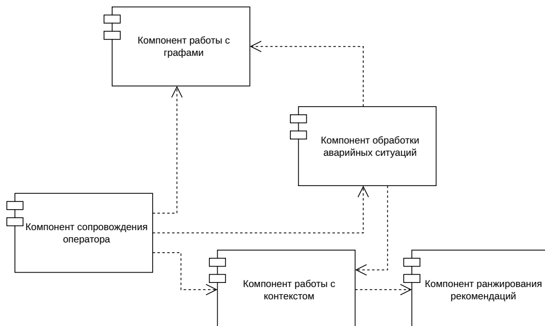
Рисунок 2.7 – Диаграмма компонентов
