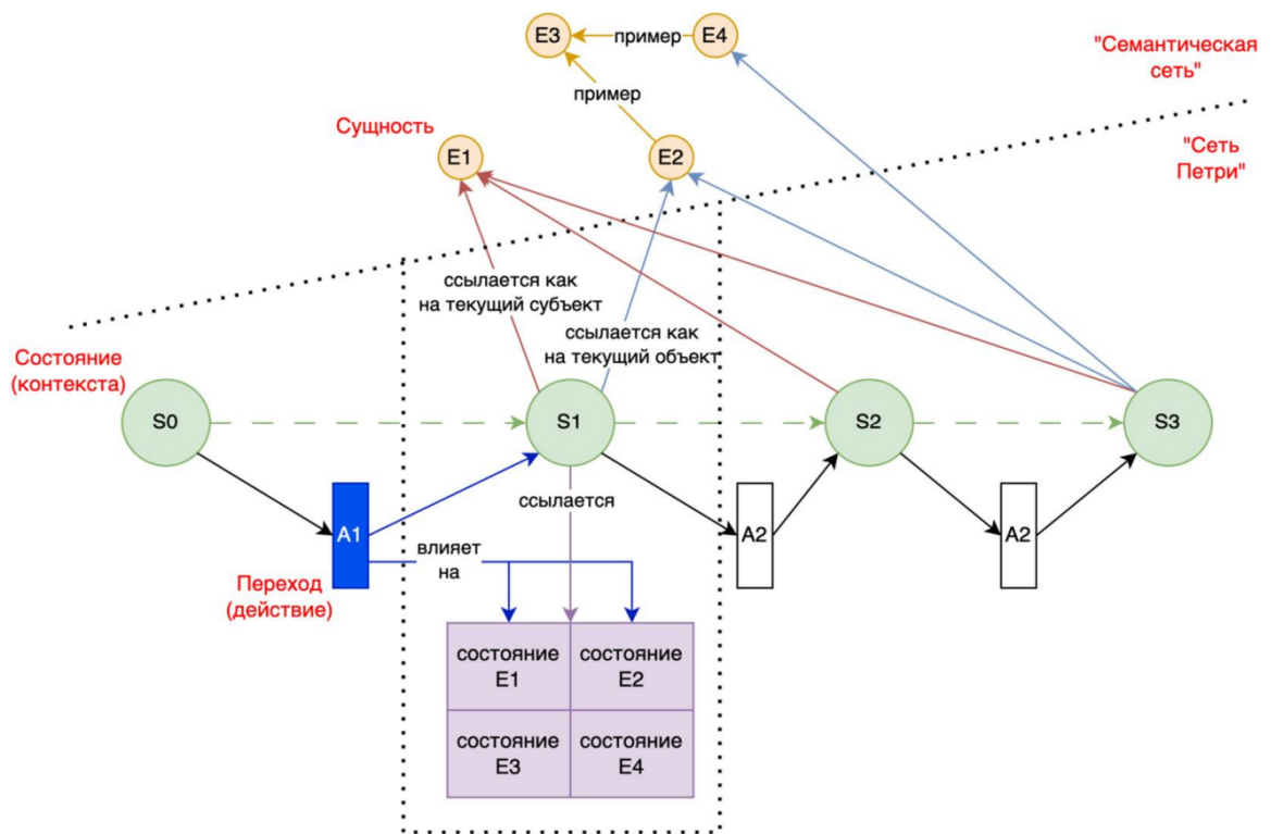
Рисунок 1.3 – Граф, описывающий инструкцию [11]
