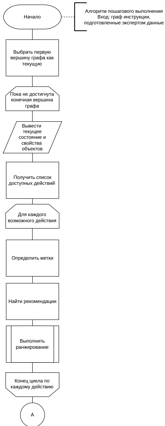
Рисунок 2.5 – Схема алгоритма пошагового выполнения, часть 1
