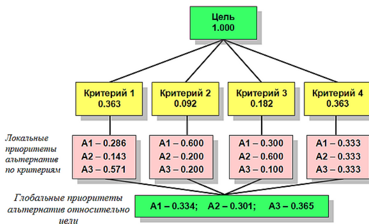
Рисунок 1.5 – Иерархическая структура МАИ с приоритетами [14]
