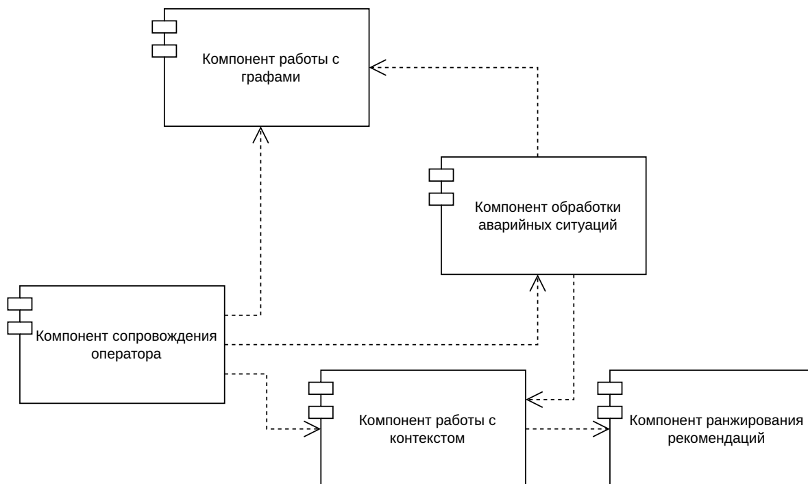
Рисунок 2.7 – Диаграмма компонентов
