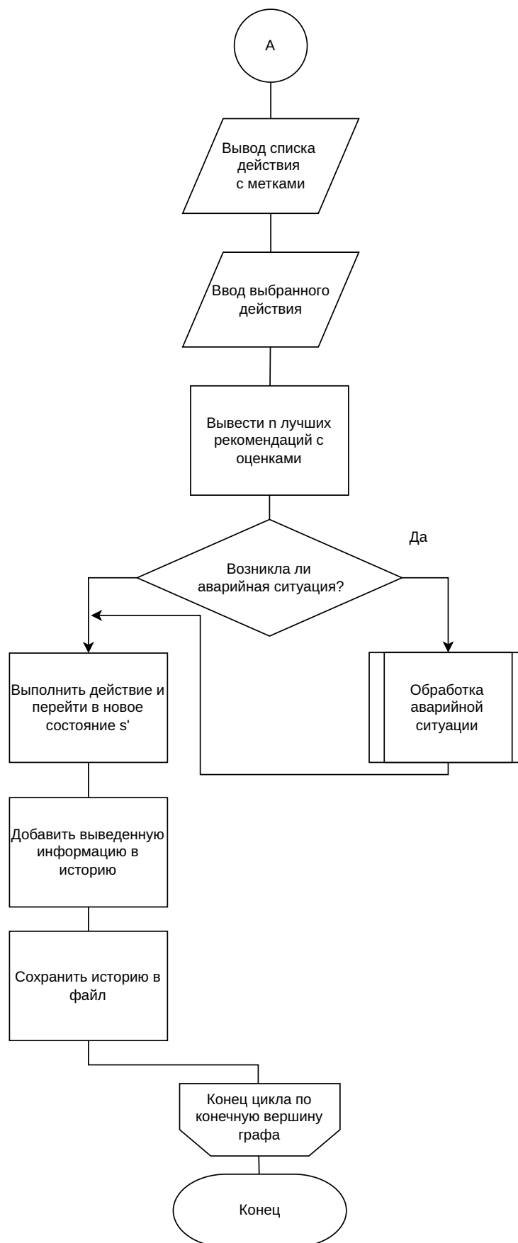
Рисунок 2.6 – Схема алгоритма пошагового выполнения, часть 2
