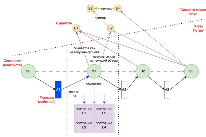
Рисунок 3.1 – Граф, описывающий инструкцию [8]
