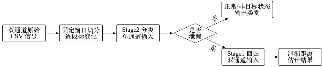
图 3-1 两阶段管道泄漏检测与定位流程
