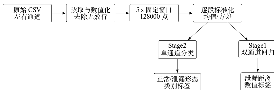
图 2-2 原始信号到监督学习样本的数据建模流程
