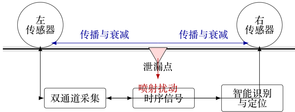
图 1-1 管道泄漏检测问题的基本物理图景
