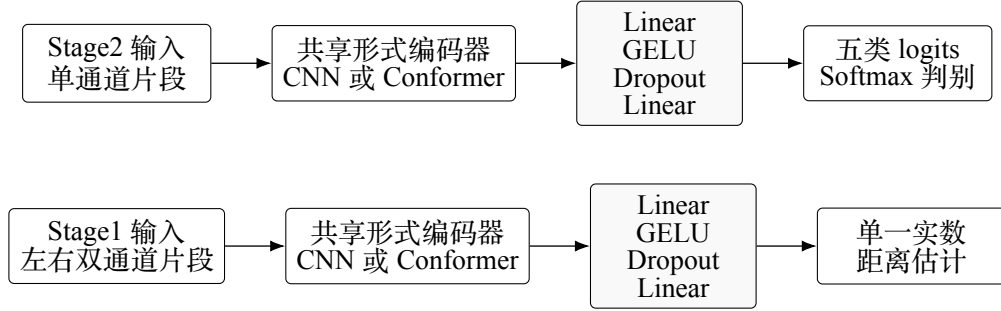
图 3-4 分类头与回归头设置示意图
