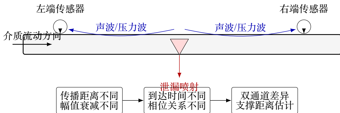
图 2-1 管道泄漏声信号传播与双通道响应差异示意图
