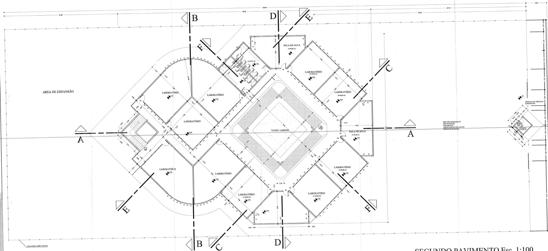
SEGUNDO PAVIMENTO Esc. 1:100
