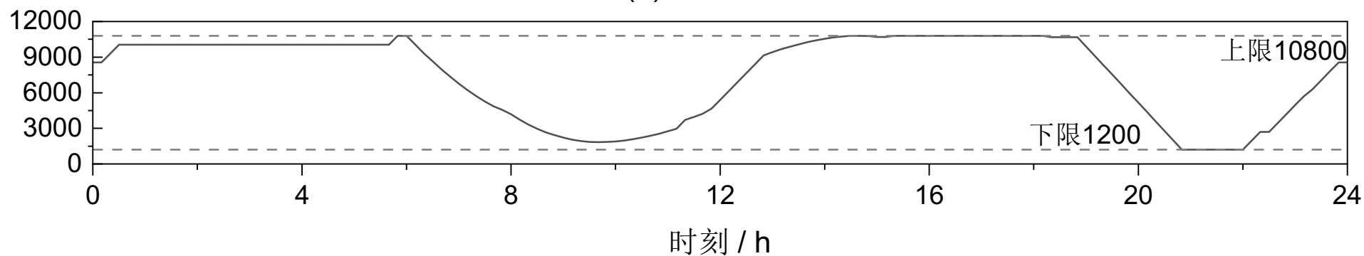
(d) 储电量轨迹
