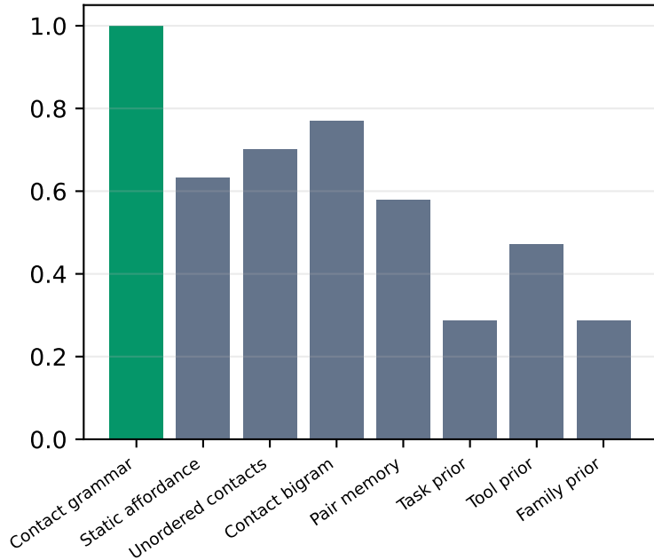
F1
