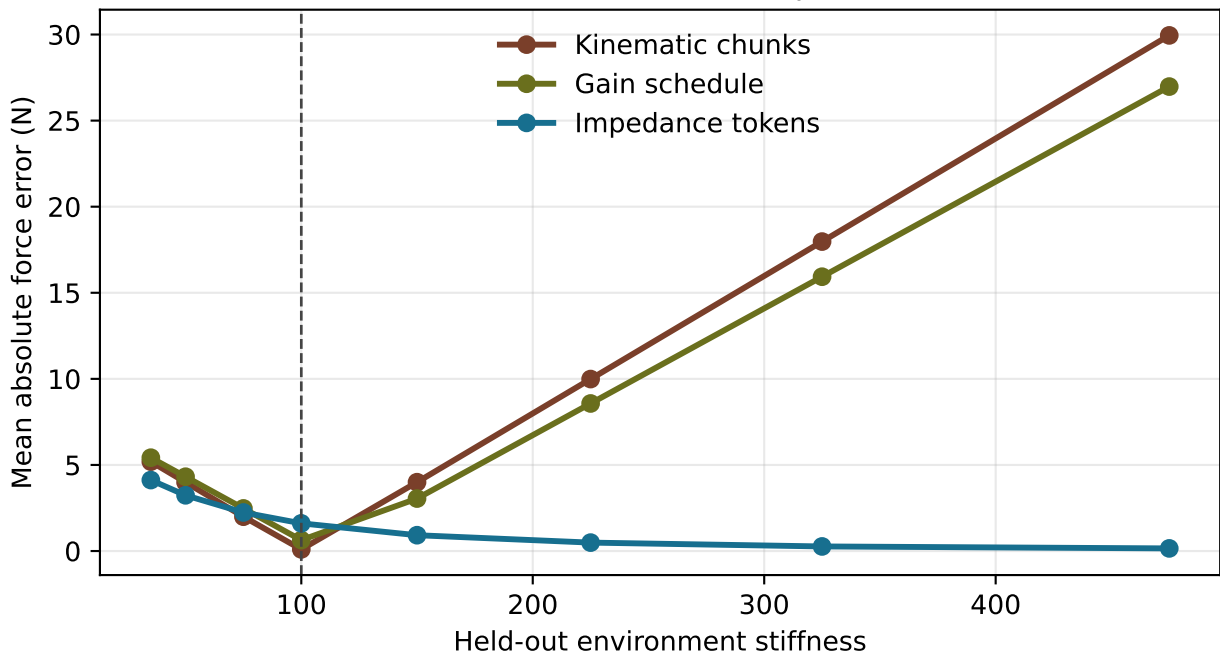
Force robustness under contact-parameter shift
