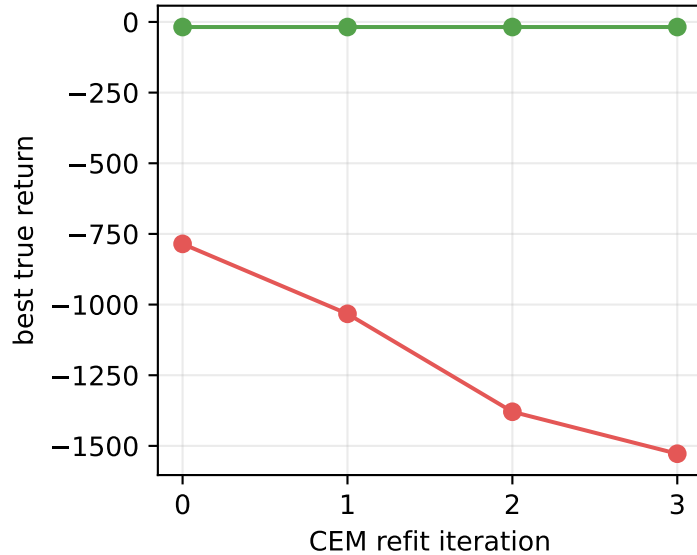
CliffWalking-v1
