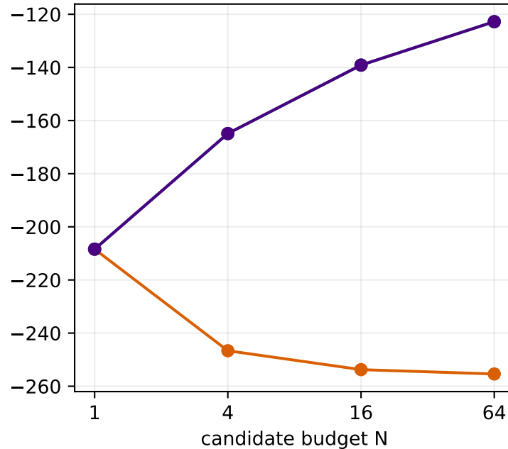
CliffWalkingSlippery-v1
