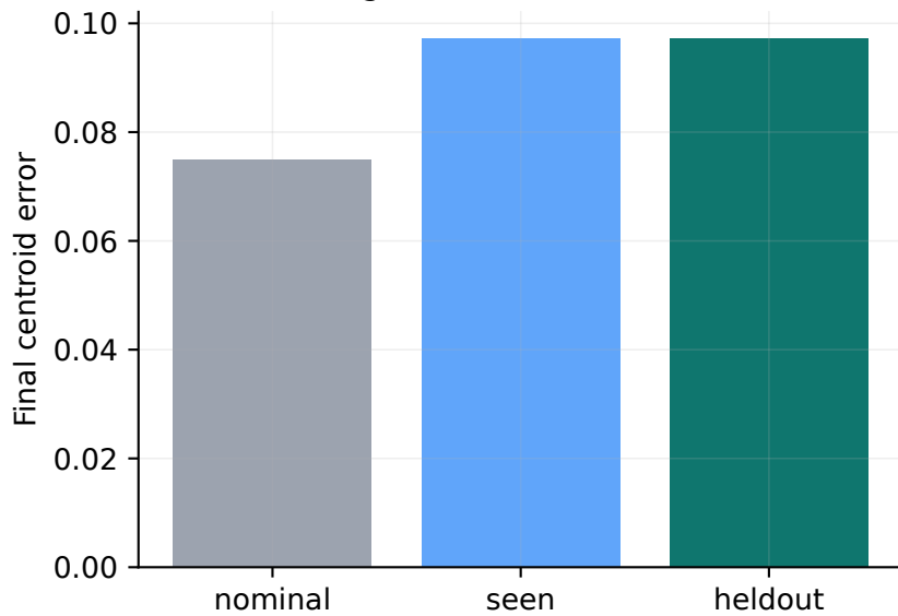
Autoregressive visual rollout drift
