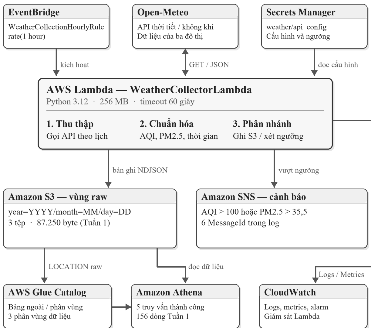
Hình 1.1. Luồng xử lý của hệ thống theo mã nguồn và cấu hình AWS
