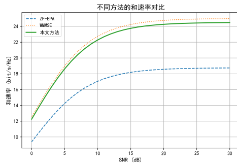
图 2. 不同方法的和速率对比
