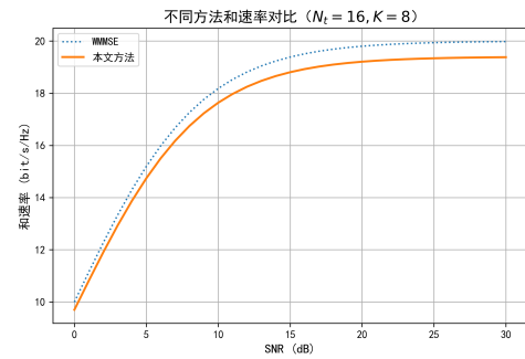
图 3. 不同方法和速率对比 ( N_t = 16, K = 8 )
