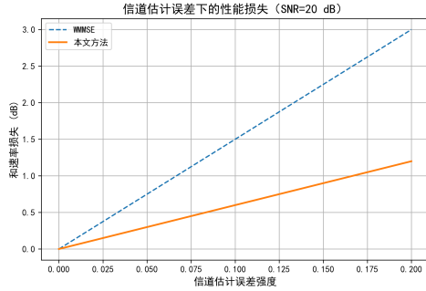
图 4. 信道估计误差下的性能损失 (SNR=20 dB)
