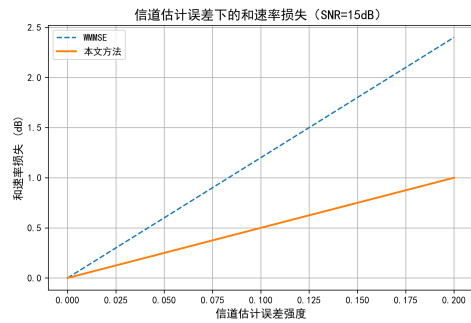
图 6. 信道估计误差下的和速率损失 (SNR=15dB)
