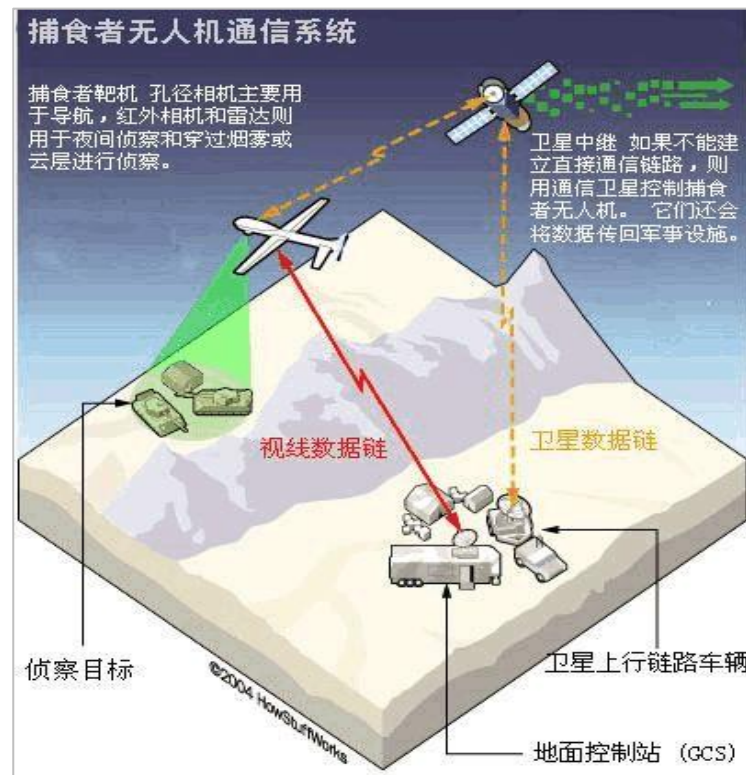
无人机通讯系统
