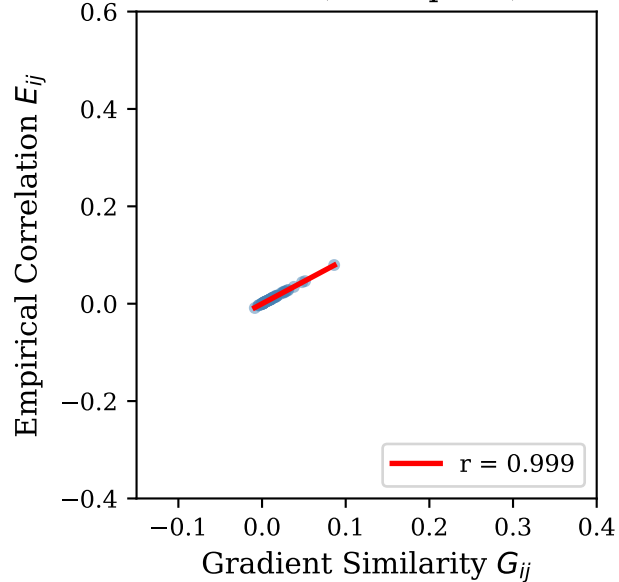
Tox21 (n=66 pairs)
