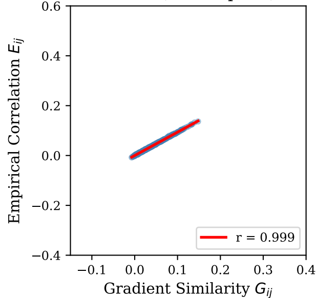
SIDER (n=351 pairs)
