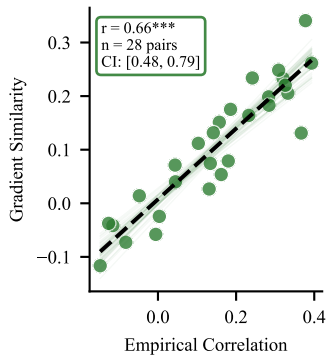
B. Within-ADME
