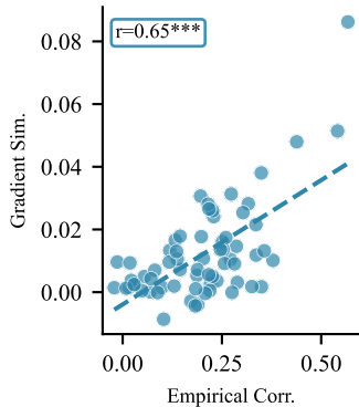
A. Tox21 (100%)
