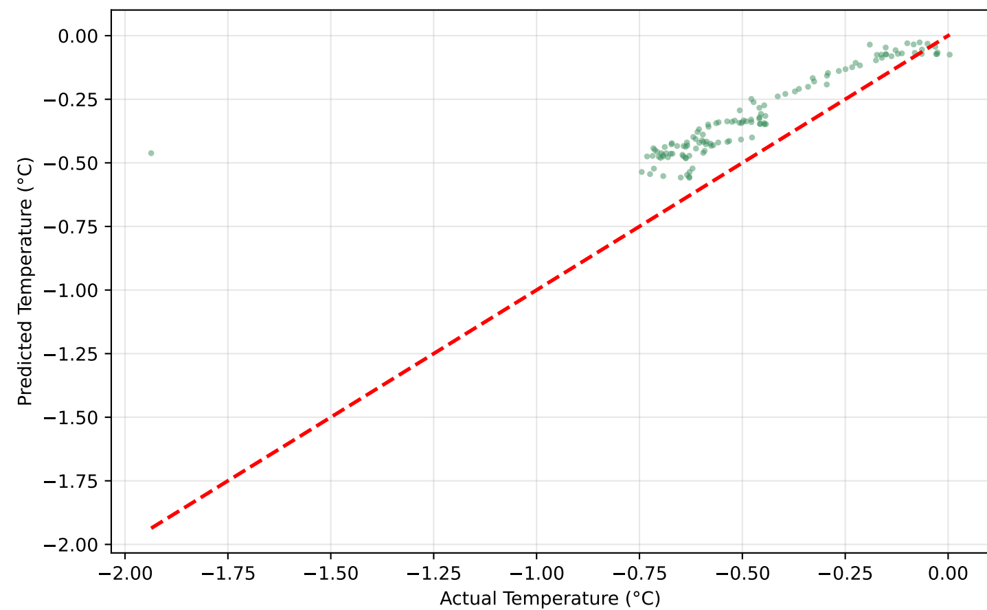
Actual vs Predicted Scatter
